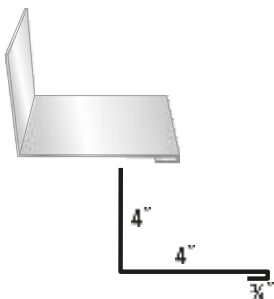
#37 SS Sidewall
