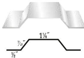
#82 Hat Channel
