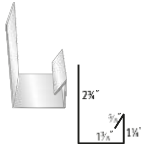
#29 Jamb Trim
